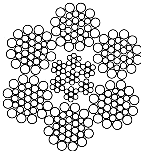
Шестипрядный канат 6 \times 31 + 1 м. с.; 6 \times 31 = 186 проволок с металлическим сердечником конструкции 7 \times 7 = 49 проволок (прядь каната 1+6+6/6+12; прядь сердечника 1+6).
